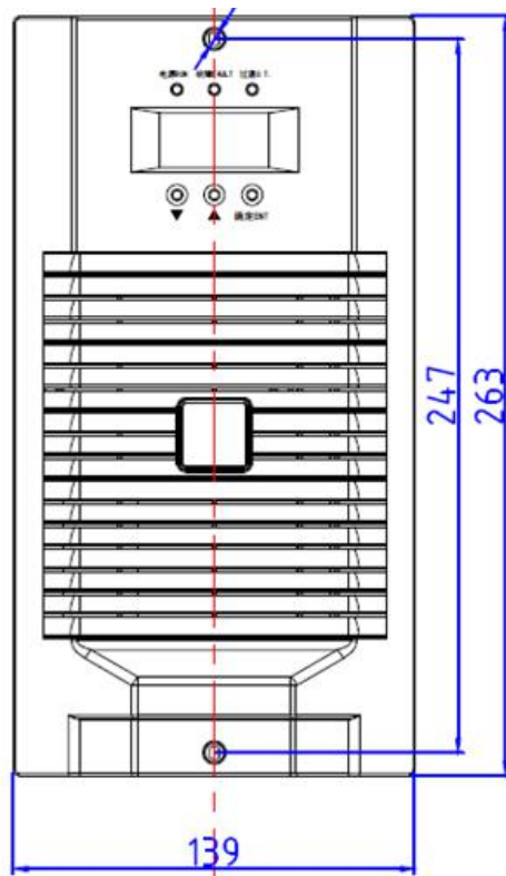
Вид спереди
